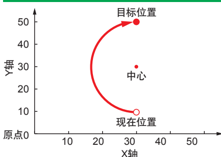
圆弧插补
