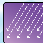
紫外线
