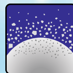
粉尘
