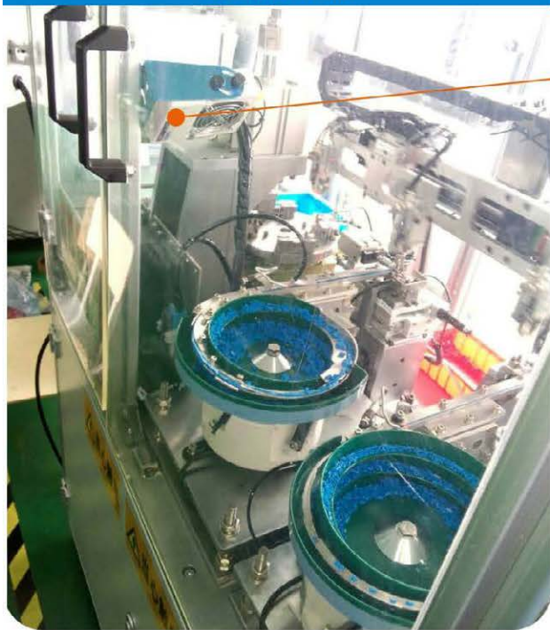
接插件组装机
