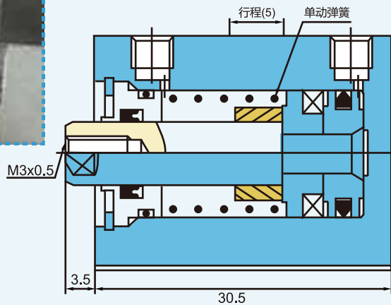
产品结构图
