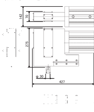
外型尺寸 MWPQ125
