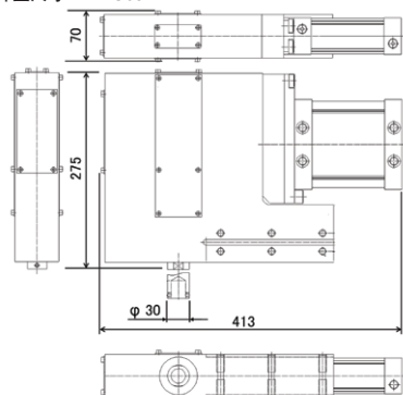
外型尺寸 MWPU63
